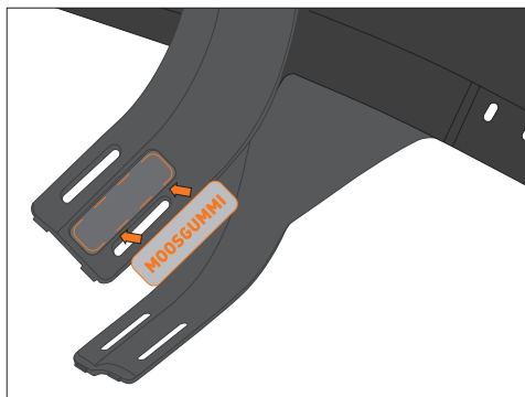
Moosgummi an Radschutz kleben (außen)
