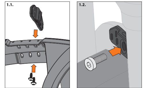
1.1. Adapter je nach benötigtem Lochbild auf dem Radschutz verschrauben. Hierfür die beiliegenden selbstschneidenden Schrauben verwenden. (TX20)
