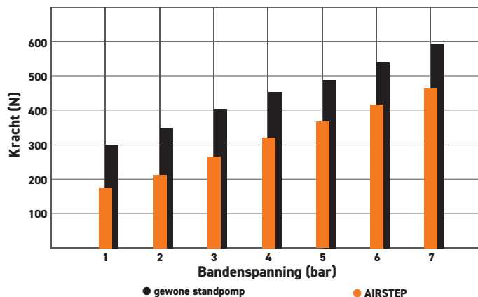
Krachtinspanning bij het pompen afhankelijk van de spanning
